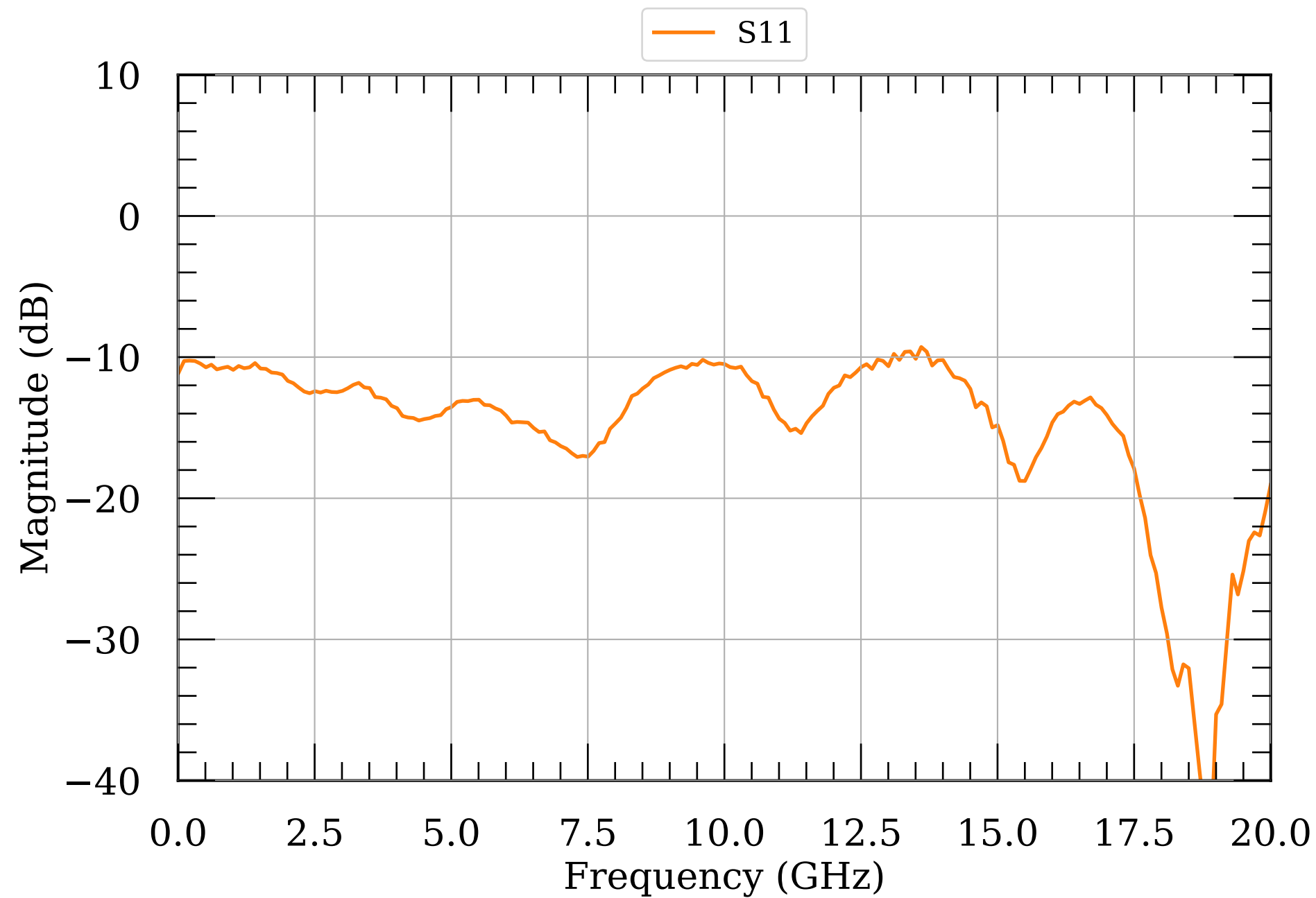
LNA S-params module085
